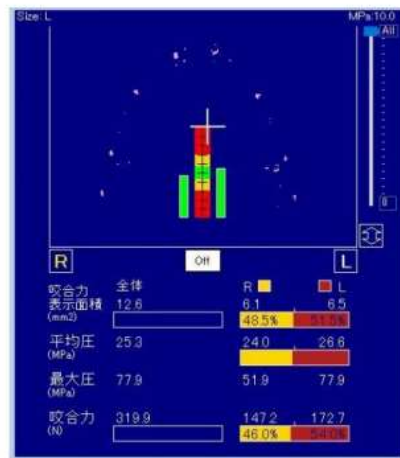
バイトフォース アナライザ(GC)
